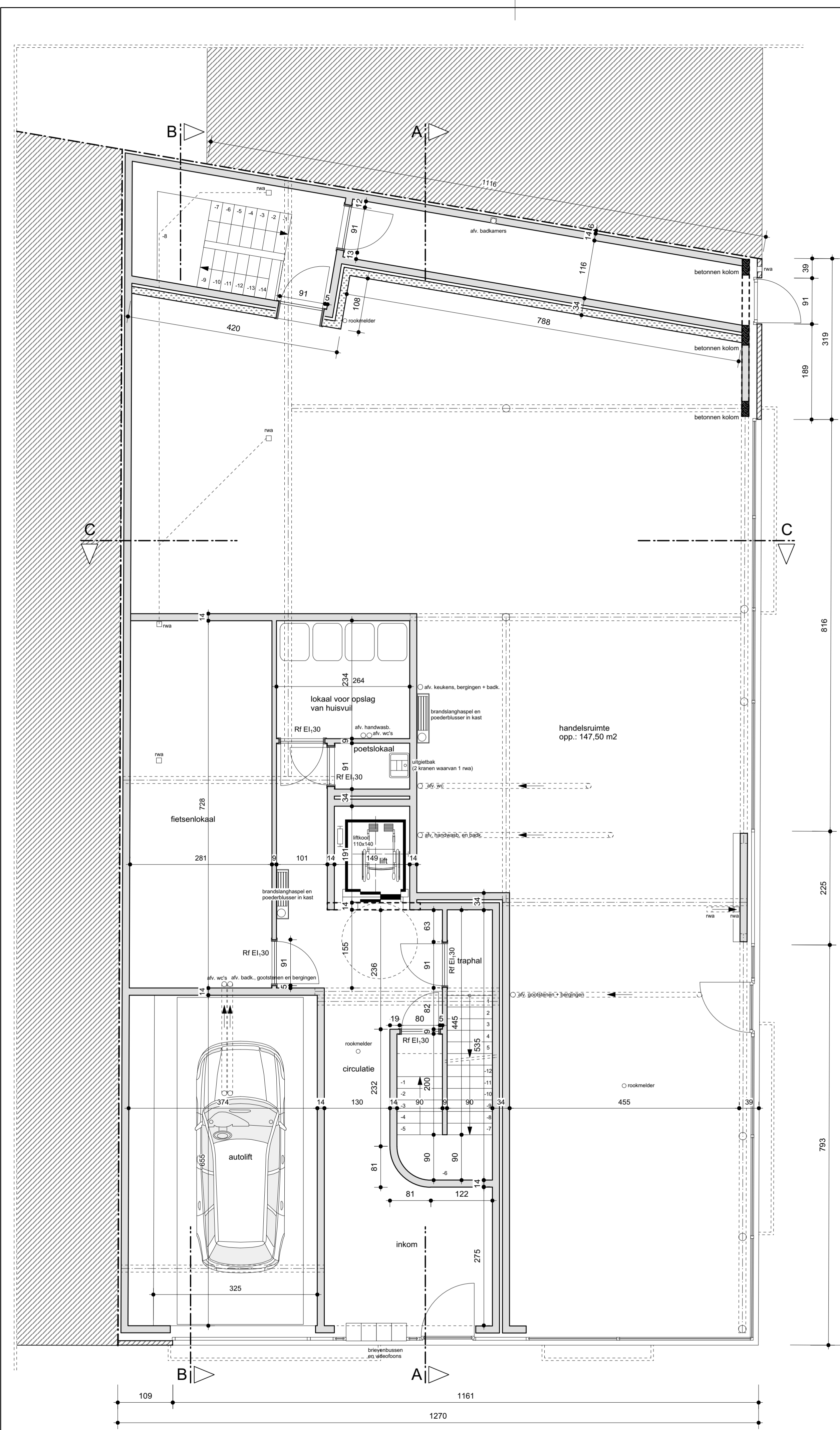
GELIJKVLOERS
