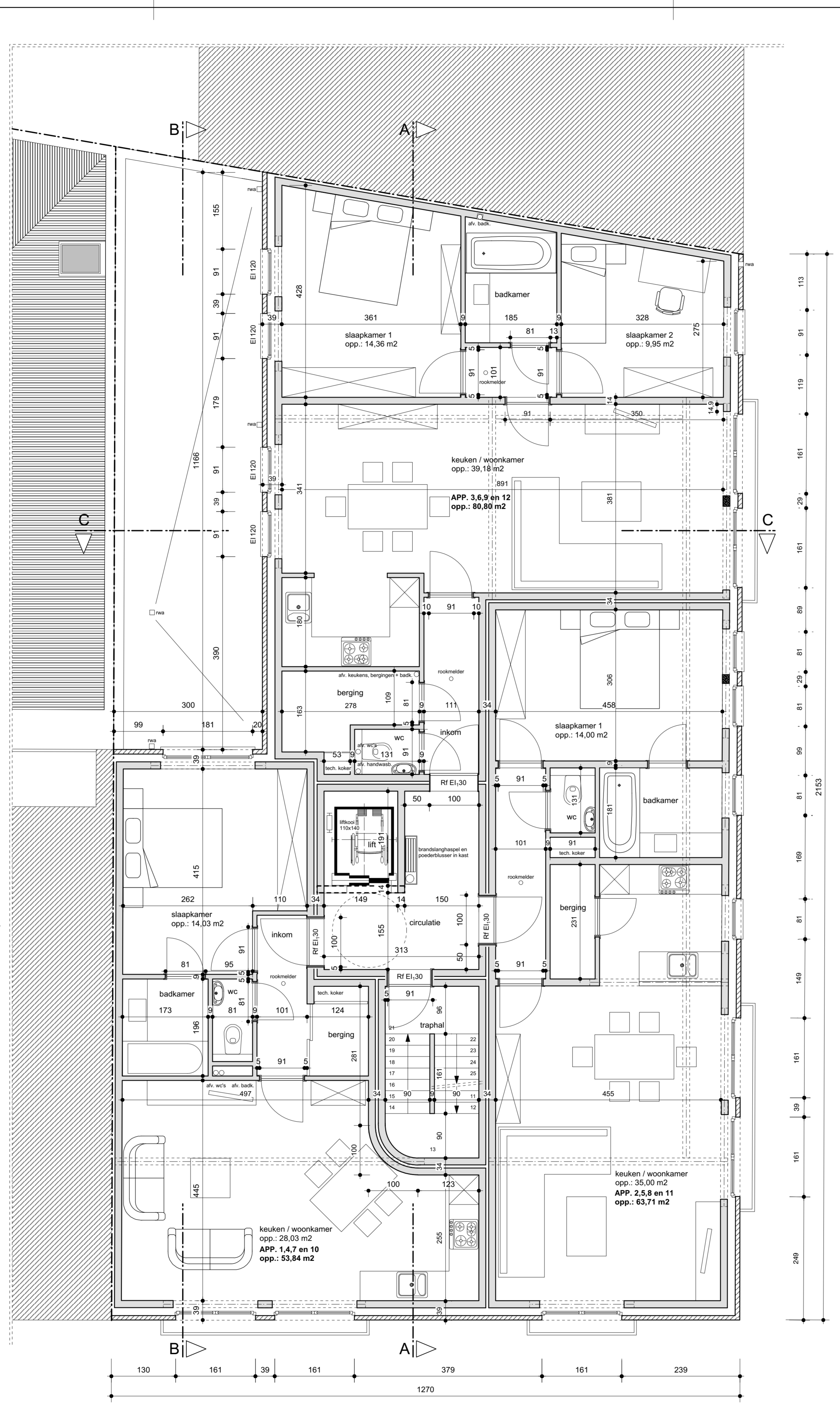
VERDIEPING 1, 2, 3 EN 4
